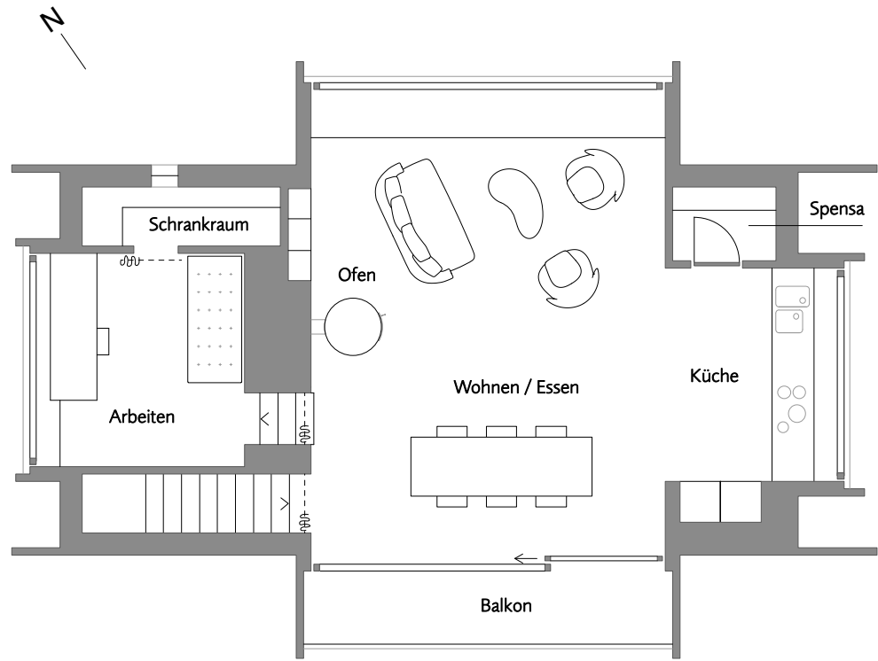
Unterhus, Zweites Obergeschoss Mst. 1:100
