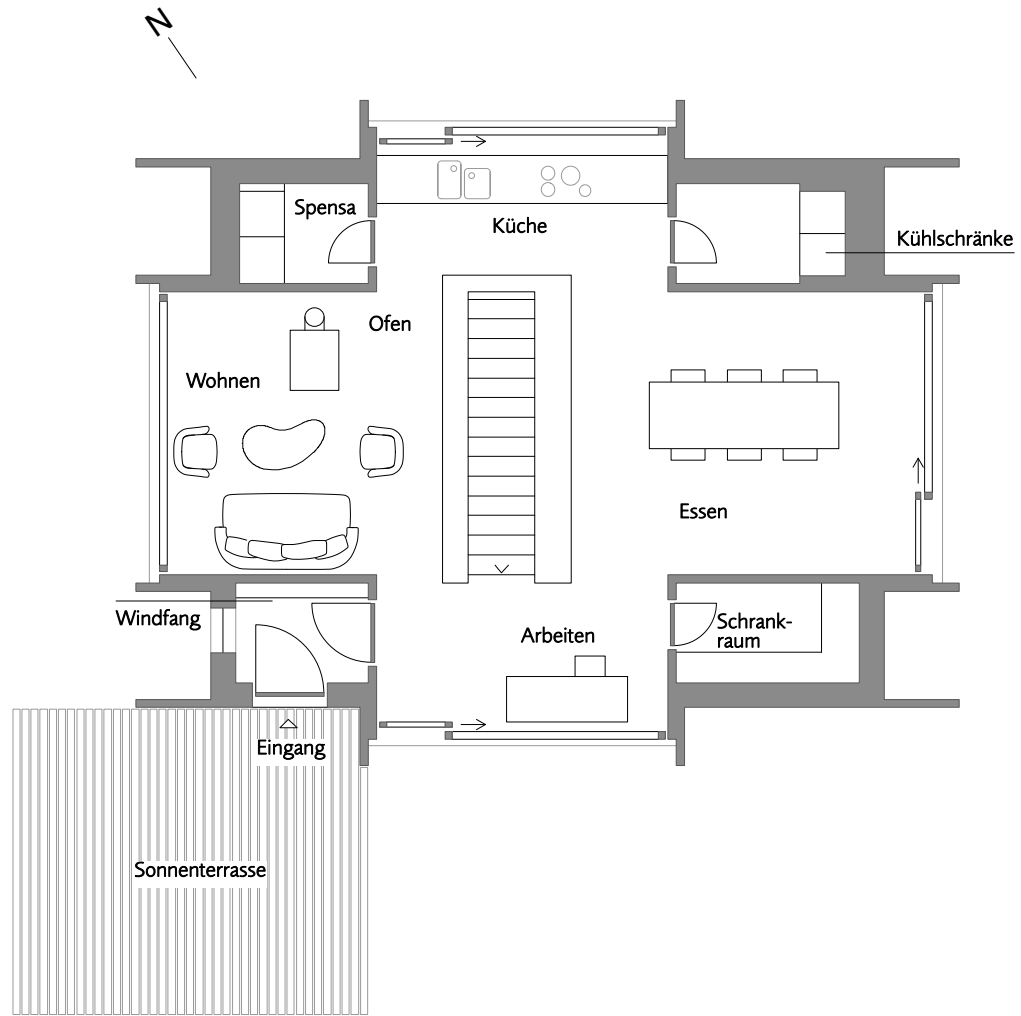
Türmlihus, Zweites Obergeschoss Masstab 1:100
