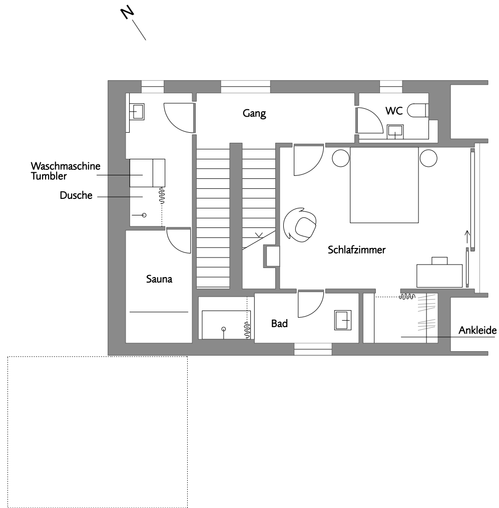
Türmlihus, Erstes Obergeschoss Massstab 1:100
